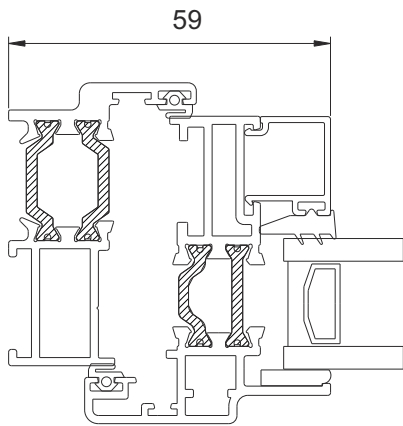
Jamb Section
