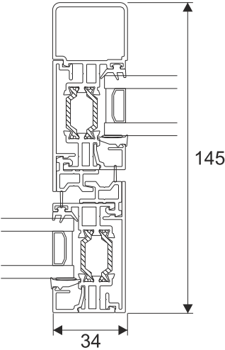
Slim Interlock
